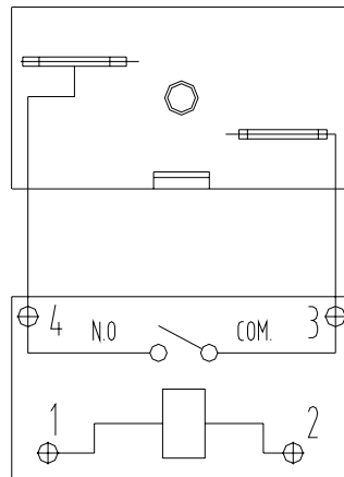
Wiring Diagram 接线图
