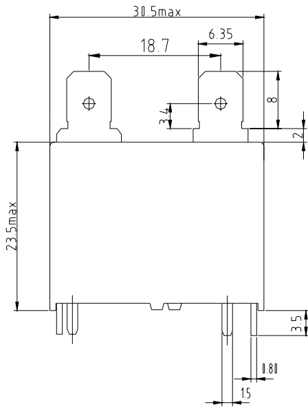
PC Board layout 安装图
