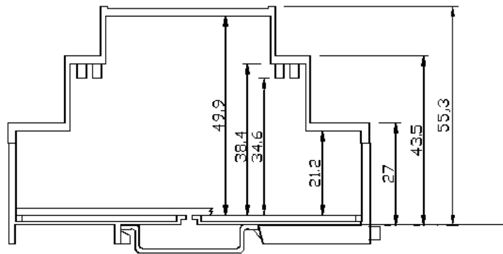
BARRA DIN
