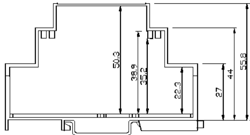
BARRA DIN
