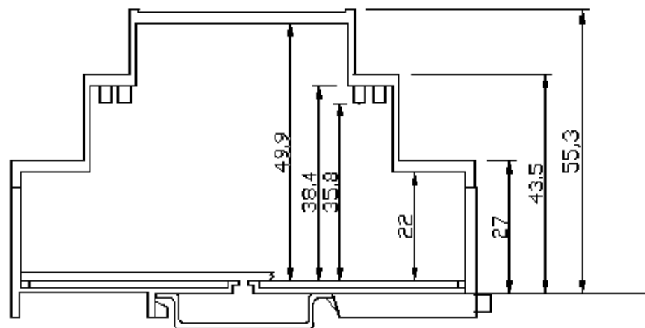
BARRA DIN
